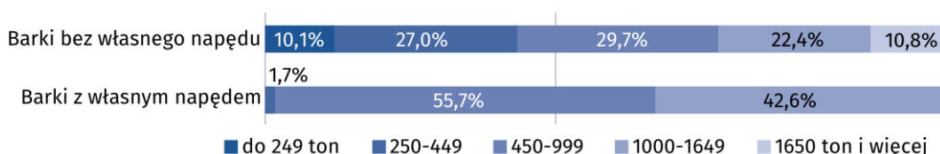
Wykres 2. Struktura taboru barkowego żeglugi śródlądowej według grup ładowności w 2022 r.
