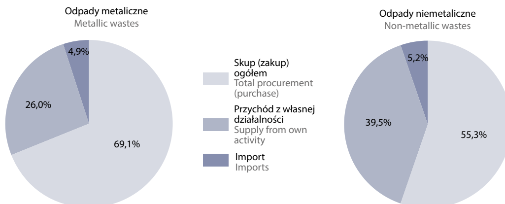
Wykres 16. Przychód ogółem odpadów nadających się do recyklingu w 2022 r. Chart 16. Total supply of wastes suitable for recycling in 2022
