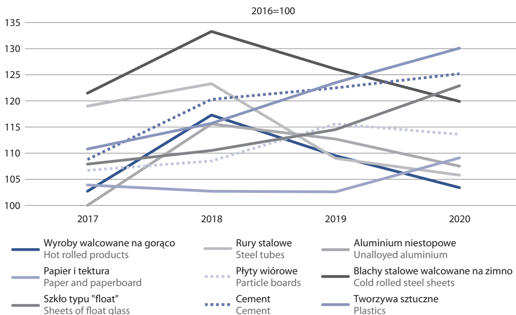
Wykres 1. Zużycie krajowe wybranych materiałów w latach 2017–2020 Chart 1. Domestic consumption of selected materials in 2017–2020
