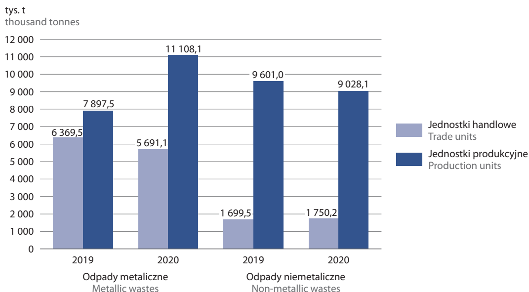
Wykres 22. Przychód odpadów nadających się do recyklingu według rodzaju jednostki w latach 2019–2020 Chart 22. Supply of wastes suitable for recycling by type of unit in 2019–2020
