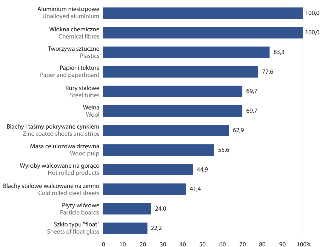
Wykres 4. Udział importu w zużyciu krajowym wybranych materiałów w 2020 r. 2 Chart 4. Share of imports in domestic consumption of selected materials in 2020
