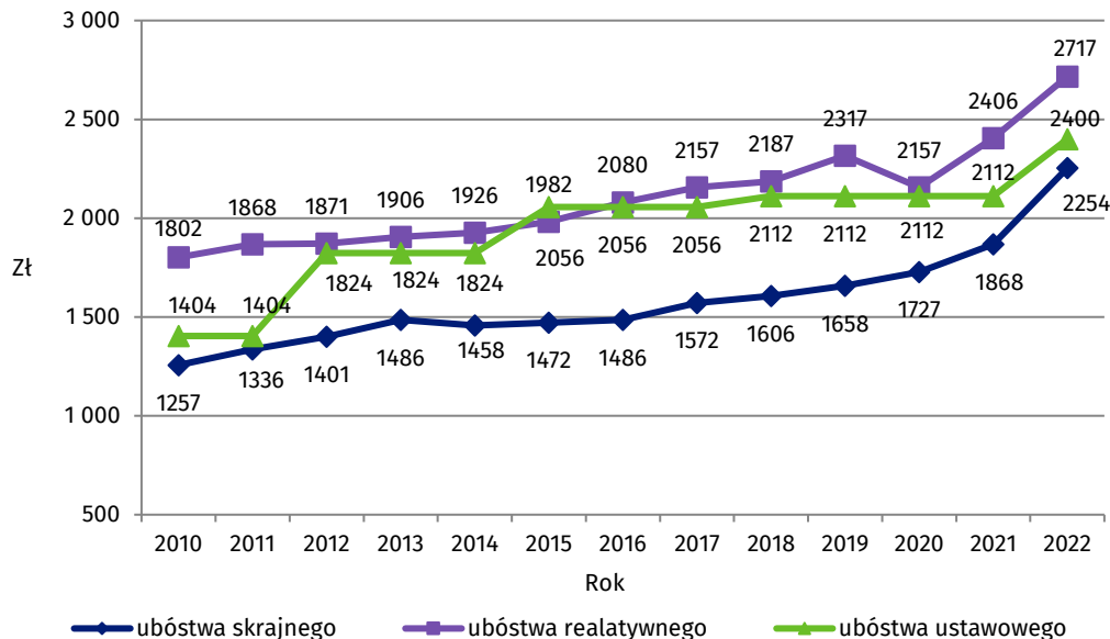
Wykres 3. Granice (progi) ubóstwa a dla gospodarstw 4-osobowych (2 osoby dorosłe + 2 dzieci do lat 14) w latach 2010–2022
