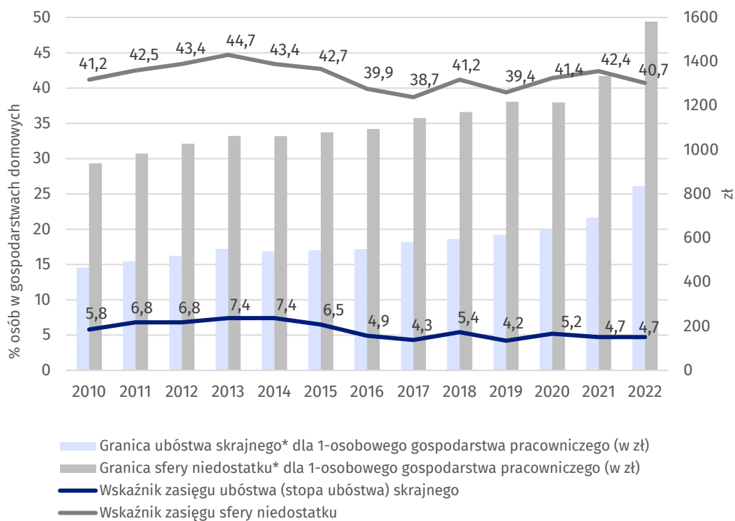
Wykres 9. Zasięg ubóstwa skrajnego oraz sfery niedostatku w Polsce w latach 2010–2022
