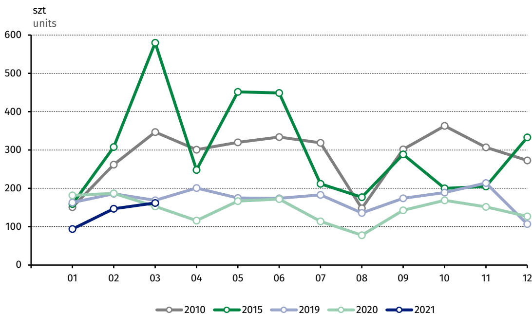
Wykres 18. Produkcja ciągników rolniczych Chart 18. Production of agricultural tractors
