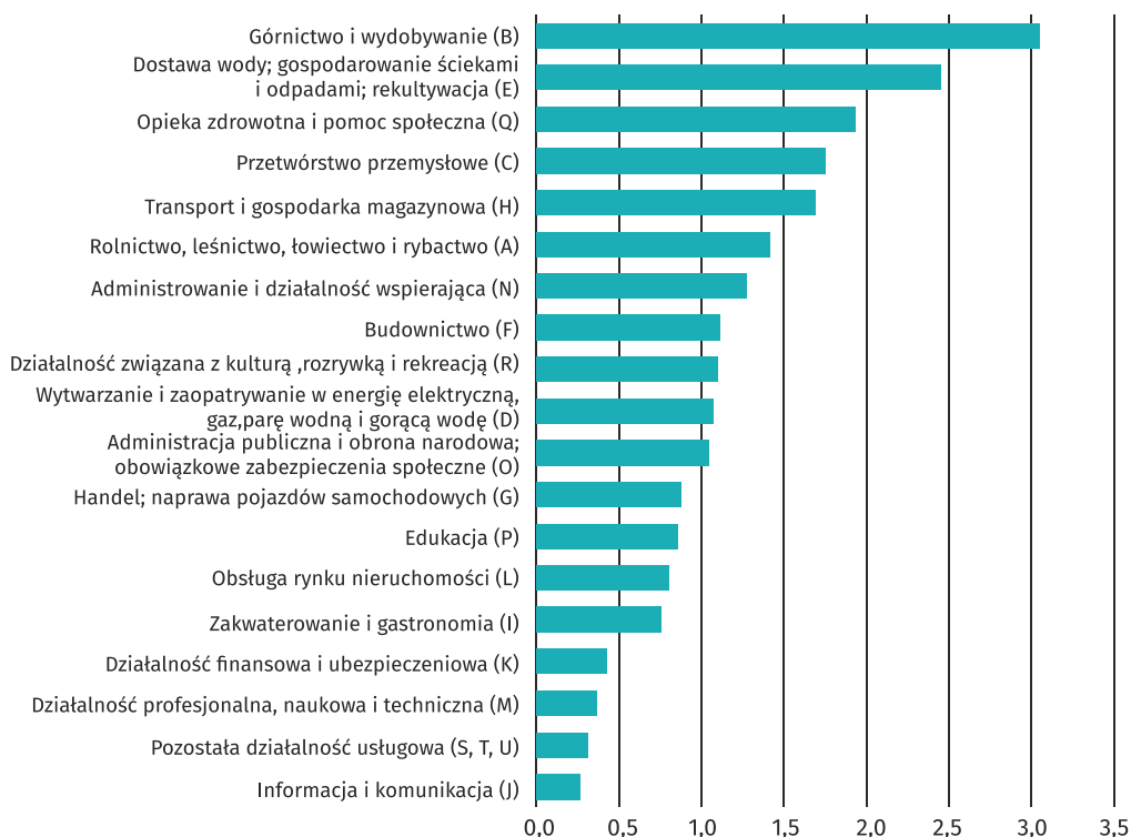
Wykres 2. Poszkodowani w wypadkach przy pracy na 1000 pracujących według sekcji PKD (bez gospodarstw indywidualnych w rolnictwie) w I kwartale 2018 r.
