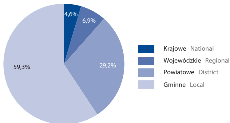
Wykres 6. Struktura dróg publicznych w 2019 r. Stan w dniu 31 grudnia Graph 6. Structure of public roads in 2019 As of 31 December
