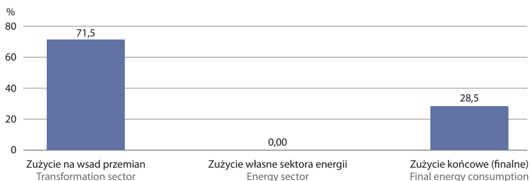
Wykres 35. Struktura zużycia biogazu w 2020 r. Chart 35. Structure of biogas consumption in 2020
