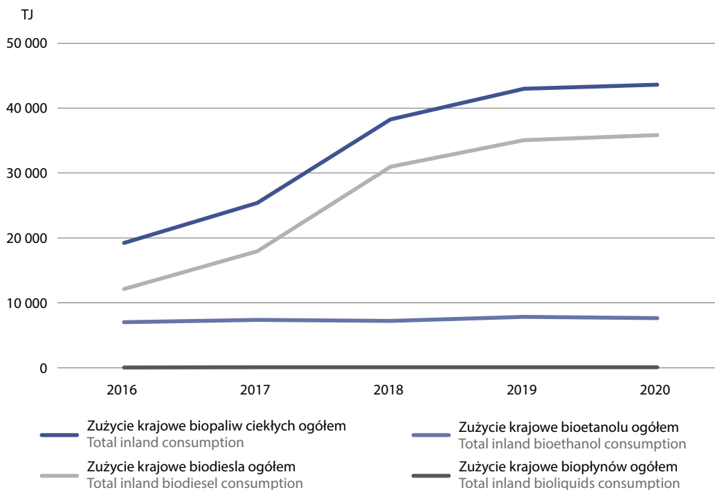
Wykres 37. Zużycie biopaliw ciekłych ogółem w latach 2016–2020 Chart 37. Total liquid biofuels consumption in the years 2016–2020
