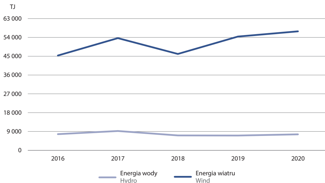
Wykres 33. Pozyskanie energii wody i wiatru Chart 33. Obtaining water and wind energy
