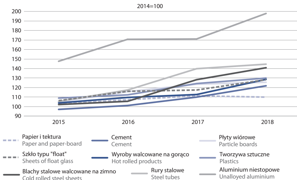
Wykres 1. Zużycie krajowe wybranych materiałów w latach 2015–2018 Chart 1. Domestic consumption of selected materials in 2015–2018
